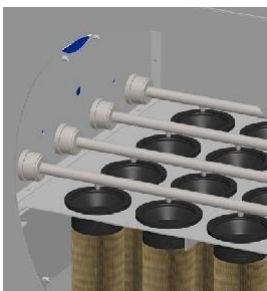
Système de rampe à dégagement rapide
